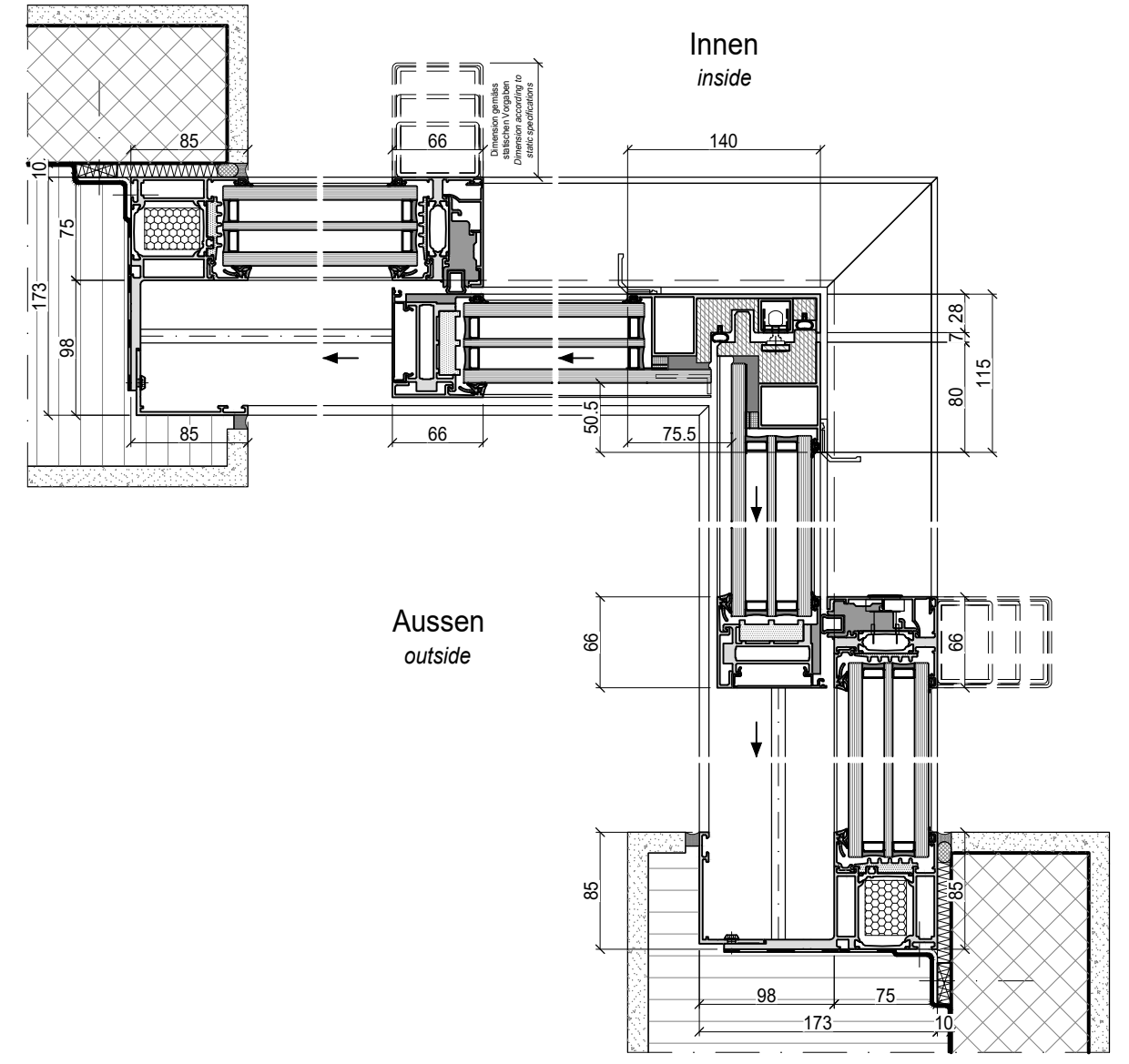
C-C
