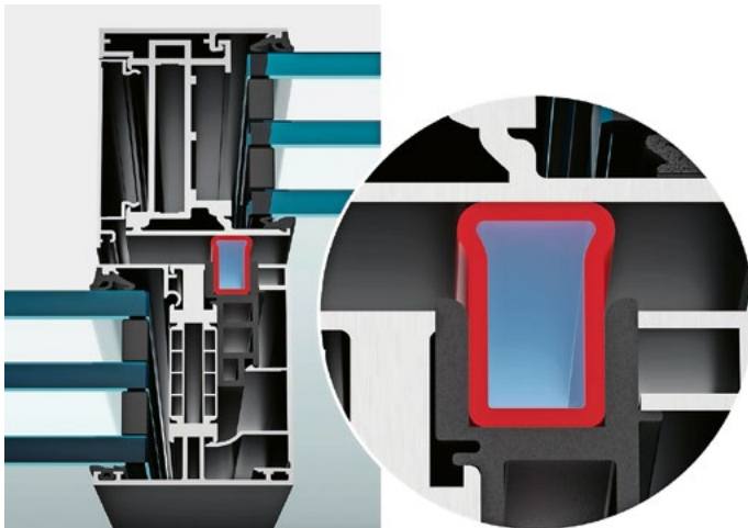
Die Dichtung drückt sich durch Knopfdruck an das Schieberprofil und verschliesst den Spalt zwischen Schieber und festem Rahmen.
